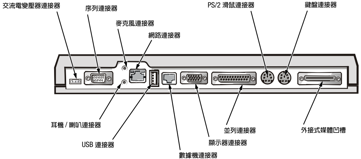
圖 3-1：將外接式裝置連接至 APR
